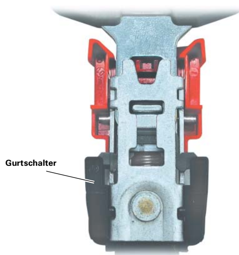
Gurtschalter gegurtet
